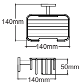
68003 Soap holder 皂篮 材质: 不锈钢 表面: 铬色
