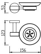
62302 Soap holder 皂碟 材质: 铜 + 不锈钢 表面: 拉丝金 + 雅黑
