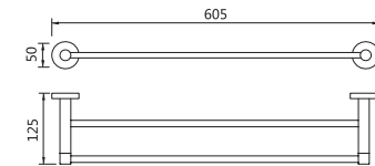
7011-B Double towel bar 双杆毛巾架 材质: 不锈钢 表面: 雅黑
