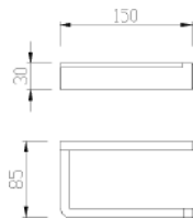
66518 Tissue holder 纸巾架 材质: 304 表面: 雅白
