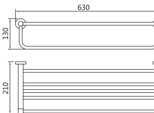
7012 Towel shelf 浴巾架 材质: 铜 + 不锈钢 表面: 铬色
