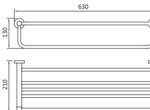
7015 Towel shelf 浴巾架 材质: 铜 + 不锈钢 表面: 铬色
