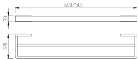
66511 Double towel bar 双杆毛巾架 材质: 304 表面: 雅白
