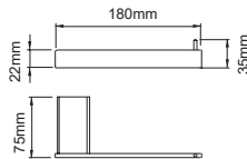
69218 Tissue holder 纸巾架 材质: 304 表面: 雅黑
