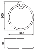
7007 Towel ring 毛巾环 材质: 铜 + 不锈钢 表面: 铬色
