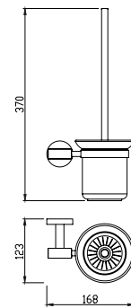
62309 Toilet brush holder 马桶刷 材质: 铜 + 不锈钢 表面: 拉丝金 + 雅黑
