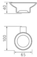
67202 Soap holder 皂碟 材质: 304 表面: 拉丝金
