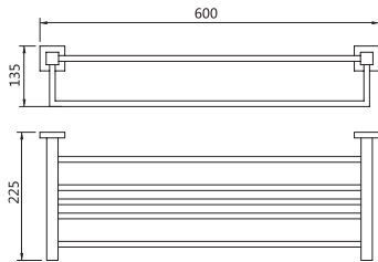
7112-M Towel shelf 浴巾架 材质: 不锈钢 表面处理: 拉丝
