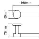
62318 Tissue holder 纸巾架 材质: 铜 + 不锈钢 表面: 拉丝金 + 雅黑
