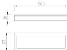
66507 Towel holder 毛巾架 材质: 304 表面: 雅白
