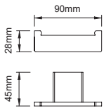
69201 Clothes hook 衣钩 材质: 304 表面: 雅黑
