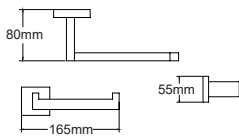
68018 Tissue holder 纸巾架 材质: 不锈钢 表面: 铬色
