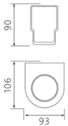
24404 Tumbler holder 单杯 材质: 锌合金 表面: 枪灰
