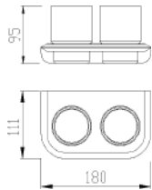
24005 Tumbler holder 双杯 材质: 锌合金 表面: 电镀
