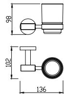
62304 Tumbler holder 单杯 材质: 铜 + 不锈钢 表面: 拉丝金 + 雅黑
