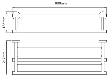
62312 Towel shelf 浴巾架 材质: 铜 + 不锈钢 表面: 拉丝金 + 雅黑
