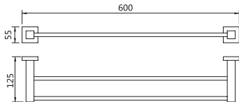
7111-M Double towel bar 双杆毛巾架 材质: 不锈钢 表面处理: 拉丝
