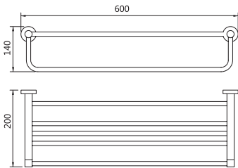
7015-B Towel shelf 浴巾架 材质: 不锈钢 表面: 雅黑
