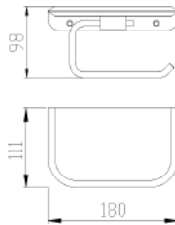
24028 Tissue holder 纸巾架 材质: 锌合金 不锈钢 表面: 电镀
