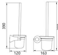
28109 Toilet brush holder 马桶刷 材质: 铜 不锈钢 表面: 金色
