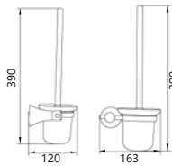
28009 Toilet brush holder 马桶刷 材质: 铜 不锈钢 表面: 铬色
