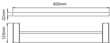
69211 Double towel bar 双杆毛巾架 表面: 雅黑
